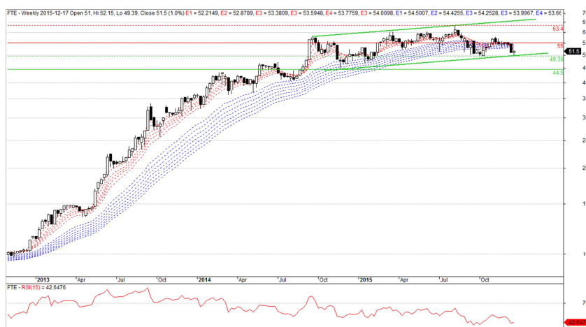
Rysunek 2. Wykres tygodniowy świecowy uwzględniający prawa z akcji.
