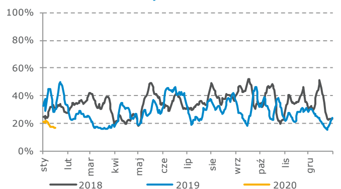
Load factor elektrowni Rybnik
