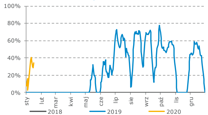
Load factor elektrowni Opole B6
