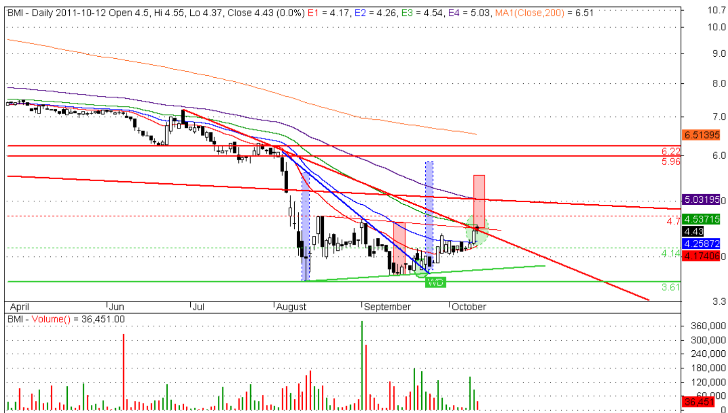
Rysunek 1. BOMI – wykres dzienny świecowy.
